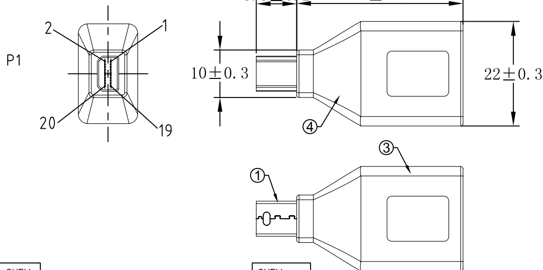
MINI DISPLAYPORT MALE
